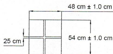
C. MESH
